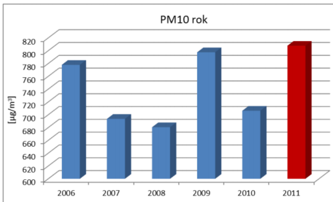
Rysunek 1-10 Stężenia średnie roczne pyłu zawieszonego PM 10 w strefie dolnośląskiej w latach 2006-2011 [źródło: Aktualizacja programu ochrony powietrza dla strefy dolnośląskiej, w której zostały przekroczone poziomy dopuszczalne pyłu zawieszonego PM 10 , tlenku węgla oraz poziomy docelowe benzo(a)pirenu i ozonu w powietrzu - projekt]
