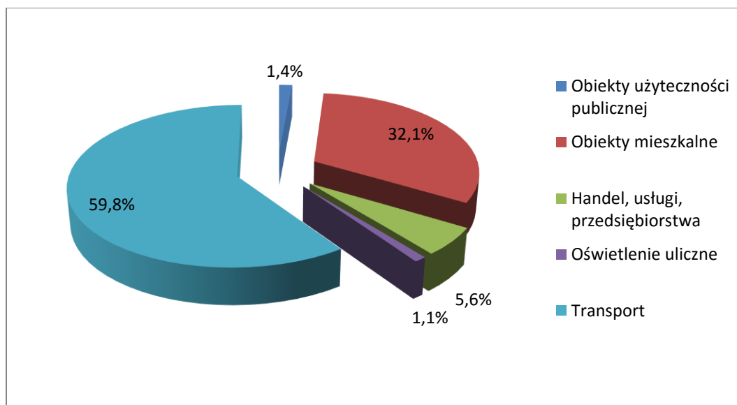
Rysunek 2-37 Udział poszczególnych sektorów odbiorców w całkowitej emisji CO 2 w roku 2020 (źródło: opracowanie własne)
